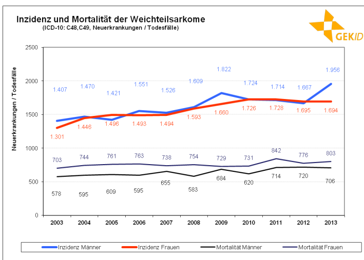
Abbildung 2: Altersstandardisierte Inzidenz und Mortalität der Weichteilsarkome in Deutschland [59]
