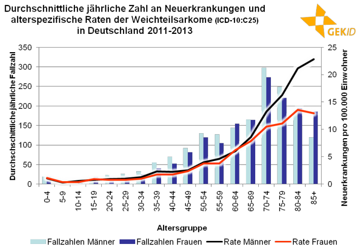
Abbildung 3: Altersspezifische Inzidenzraten und Fallzahlen [59]
