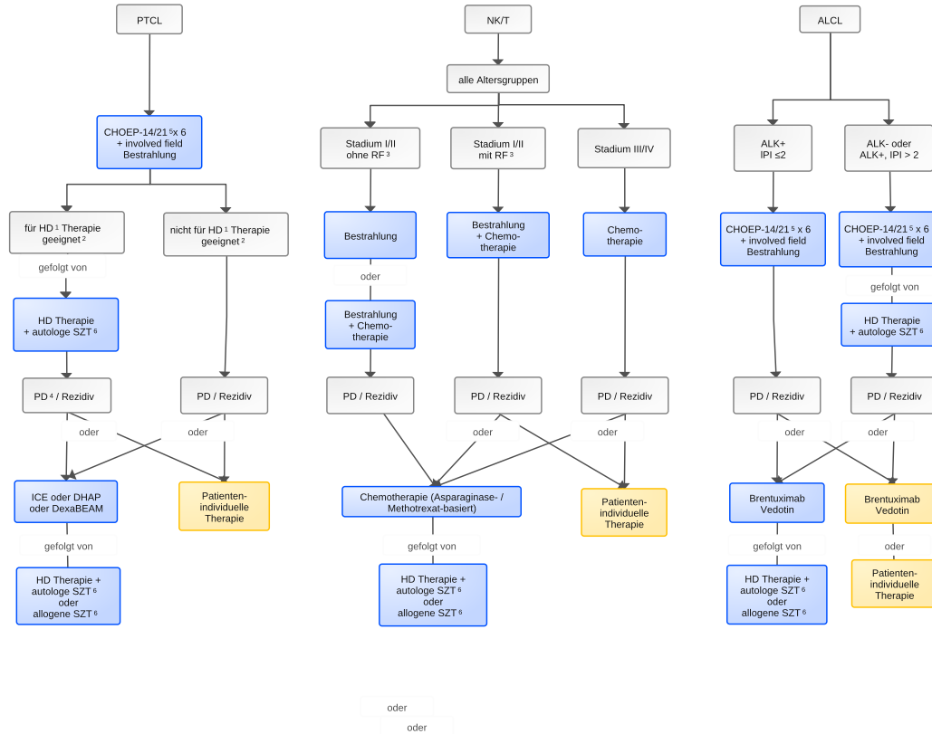
Abbildung 1: Therapiealgorithmus
